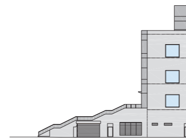
Elevation 7 立面圖 7
